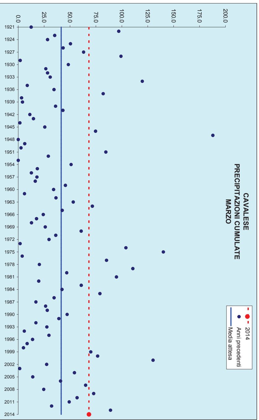
Figura 14: Precipitazioni di marzo
