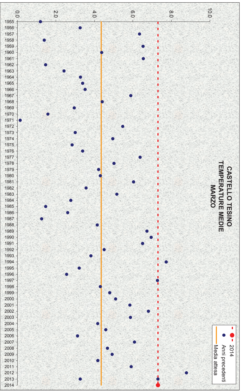
Figura 5: Temperature medie di marzo
