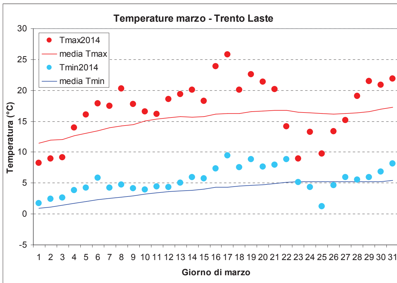
Figura 3: Temperature di marzo. La media delle Tmax e delle Tmin è riferita al periodo 1978-2005 (media mobile a 7 gg).
