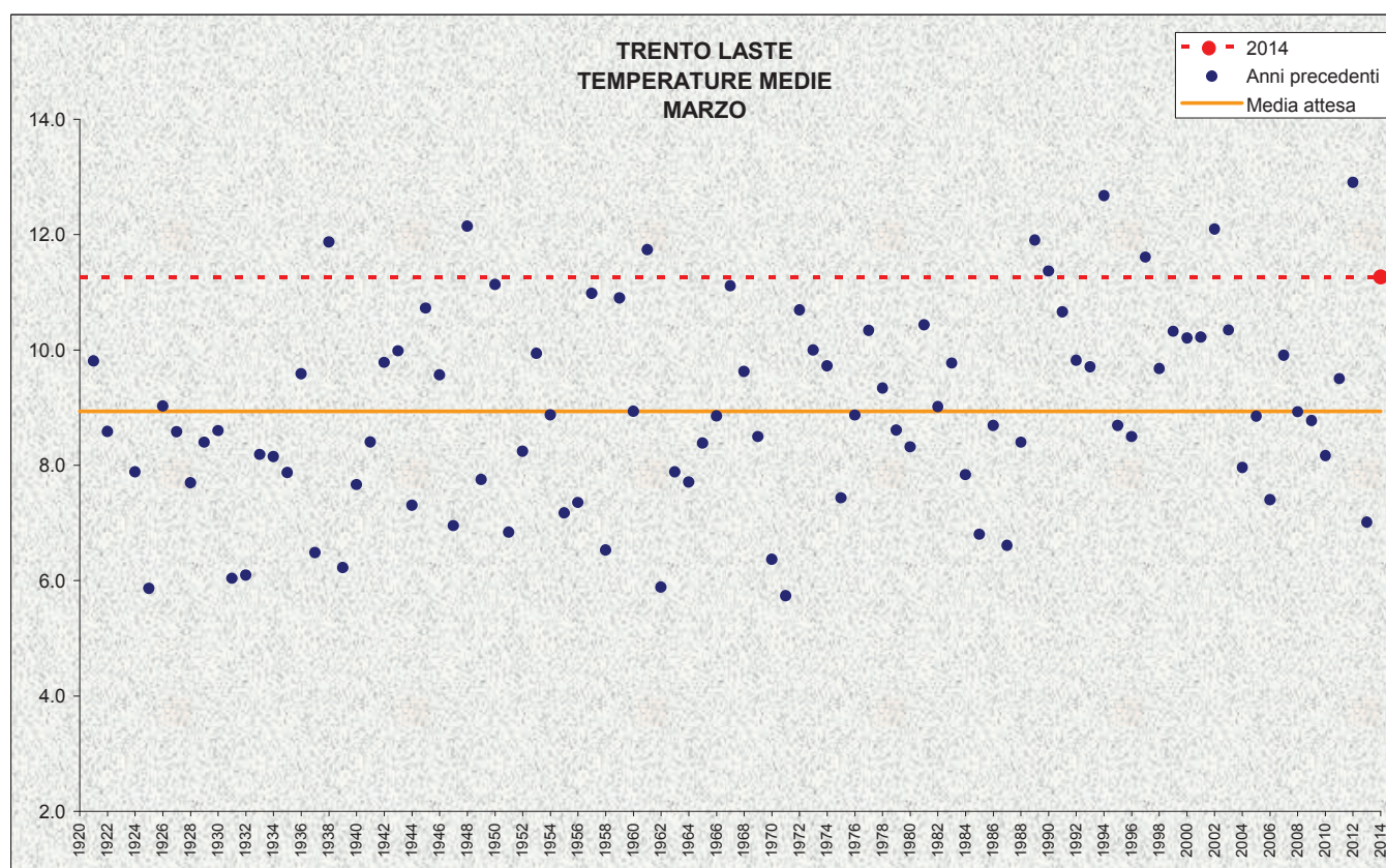
Figura 1: Temperature medie di marzo
