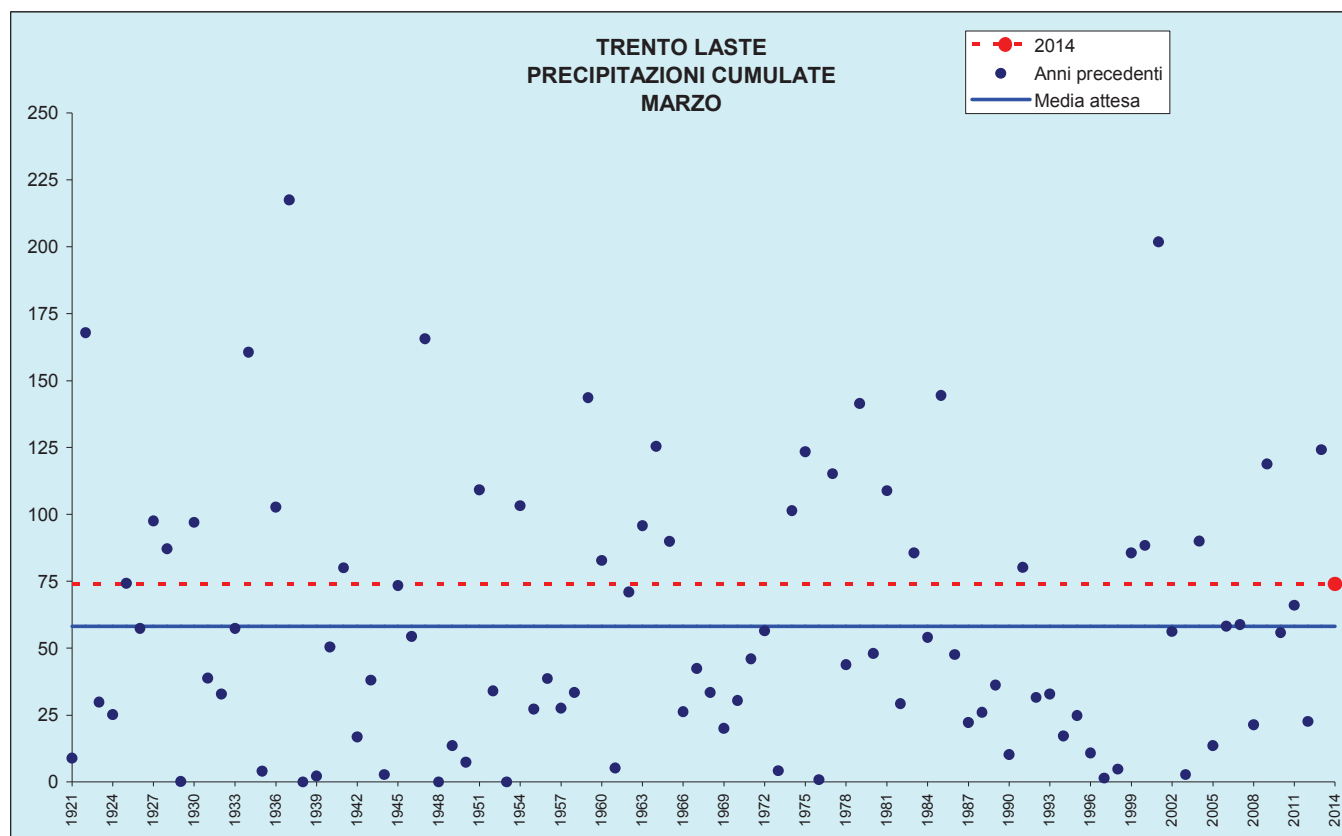
Figura 2: Precipitazioni di marzo
