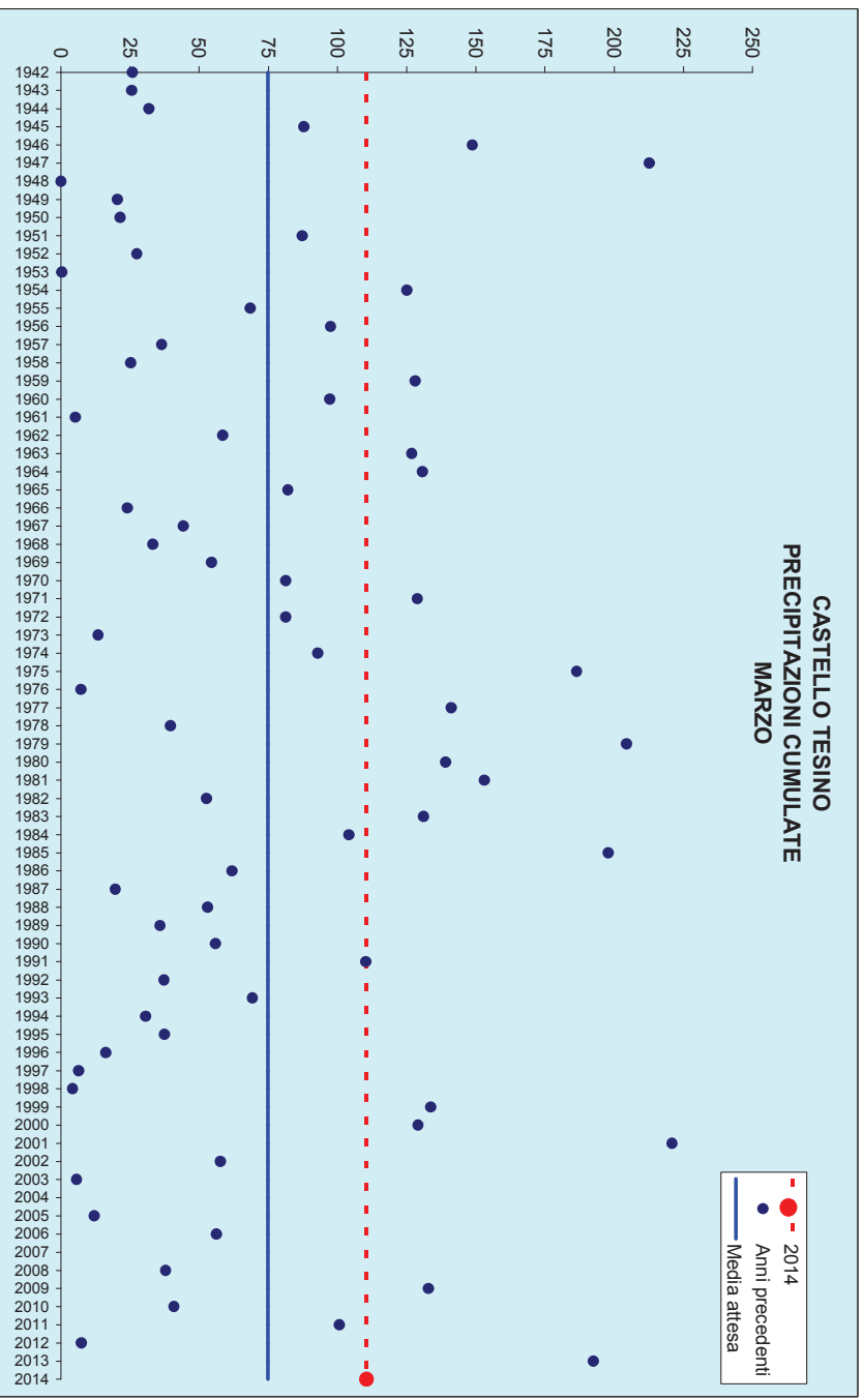
Figura 6: Precipitazioni di marzo
