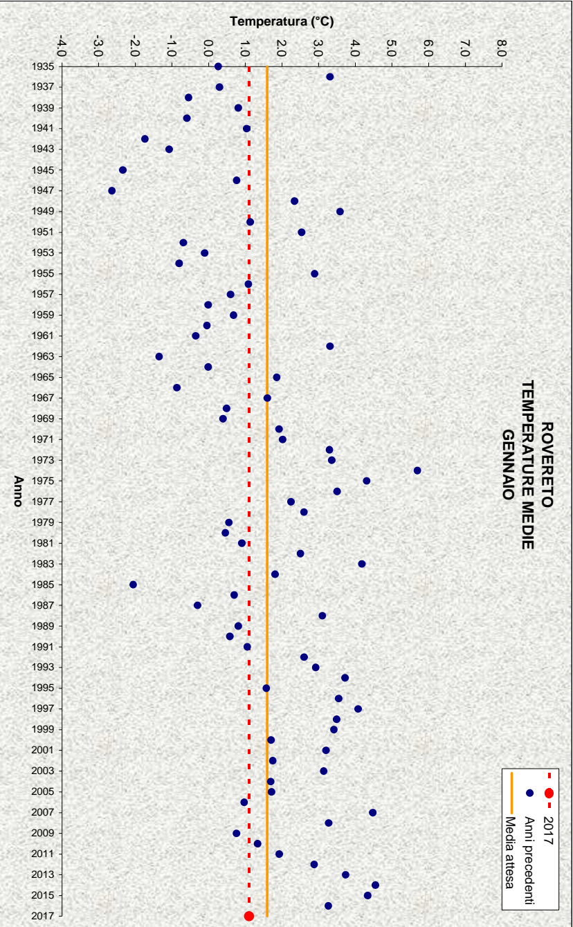
Figura 16: Temperature medie di gennaio
