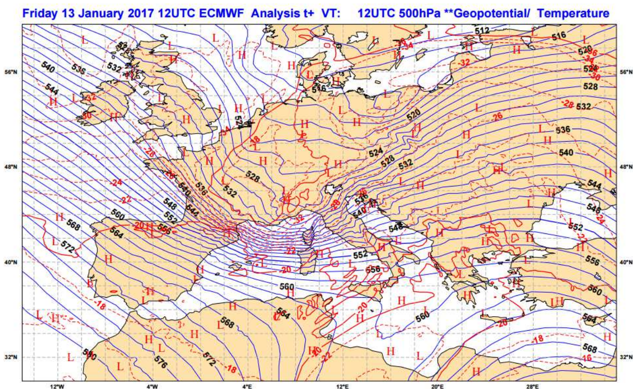
Figura 1: Analisi delle ore 12 UTC del 13 gennaio 2017 dei campi di geopotenziale e temperature della superficie 500 hPa.
