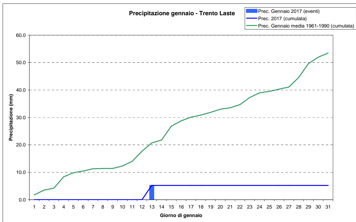
Figura 4: Precipitazioni giornaliera e cumulata di gennaio
