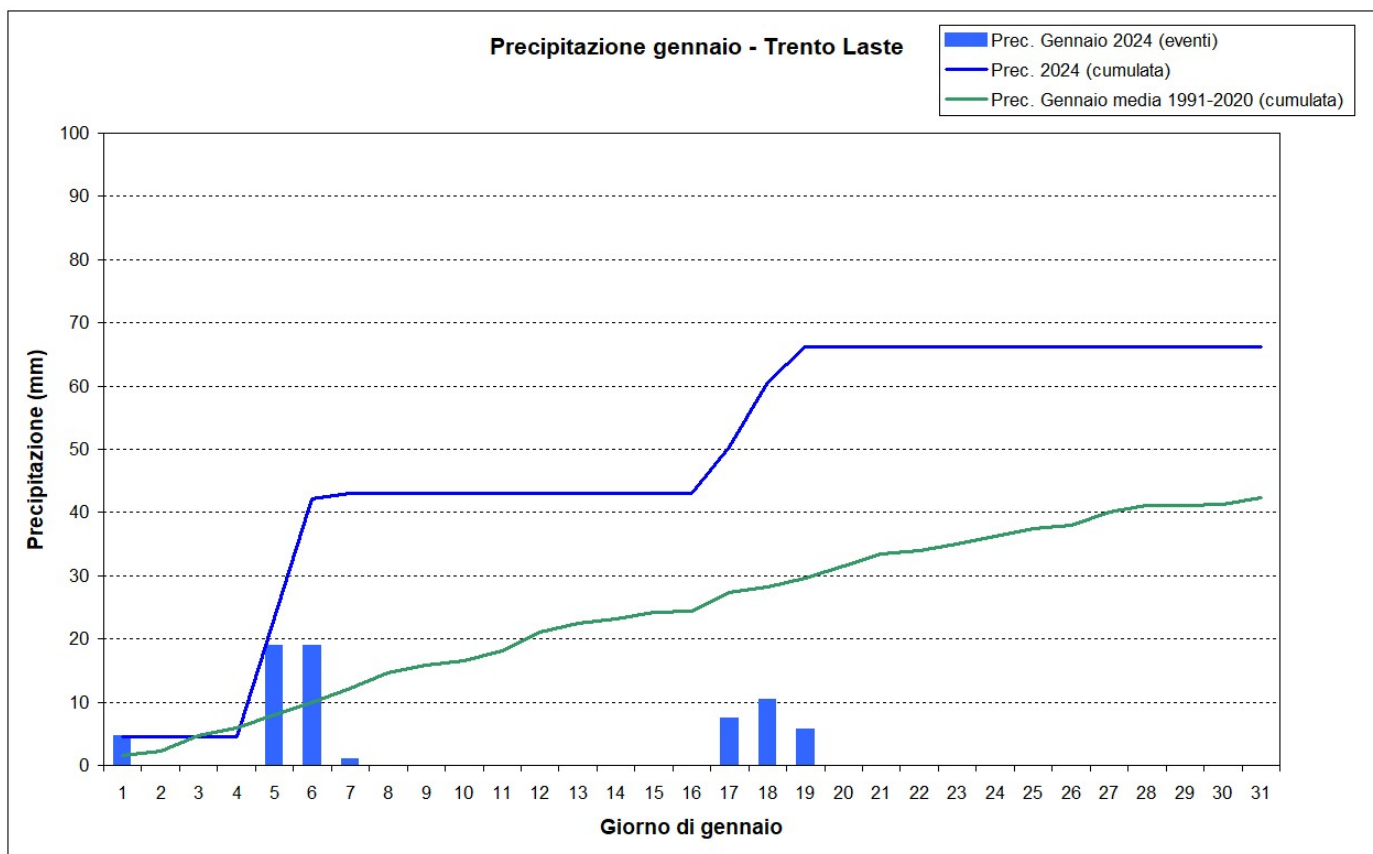
Figura 6: Precipitazione giornaliera e cumulata di gennaio (confronto con trentennio 1991-2020)
