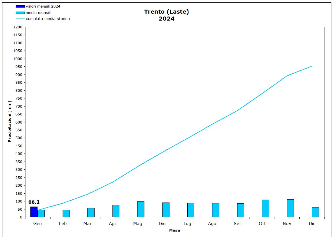
Figura 5: Precipitazione giornaliera e cumulata di gennaio
