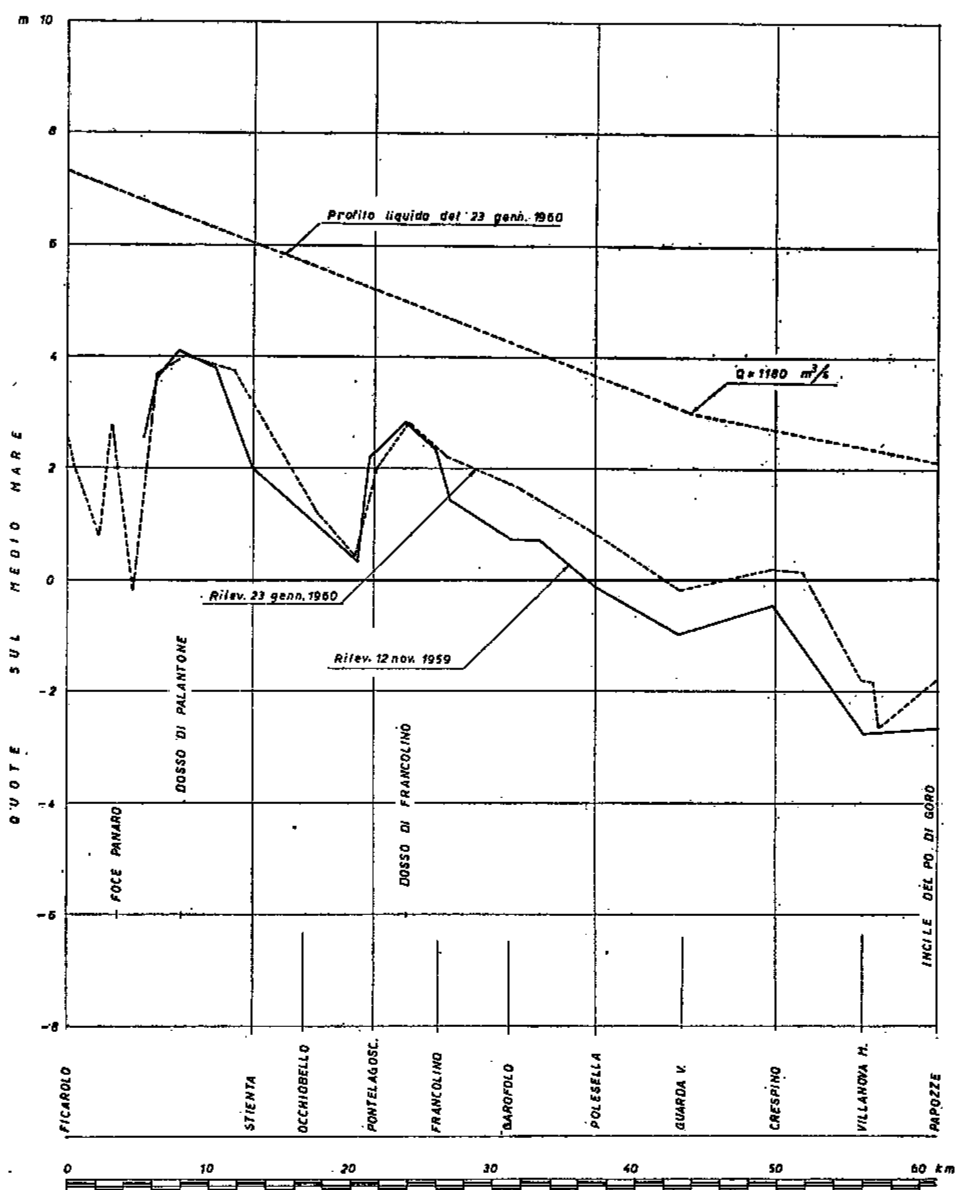
Fig. 6 — Profili involuppo dei minimi fondali nell'alveo del Po tra foce Panaro e incile Po di Goro. Linea tratteggiata: situazione di qualche mese prima e di un mese dopo la piena. Linea continua: situazione immediatamente precedente la piena.
