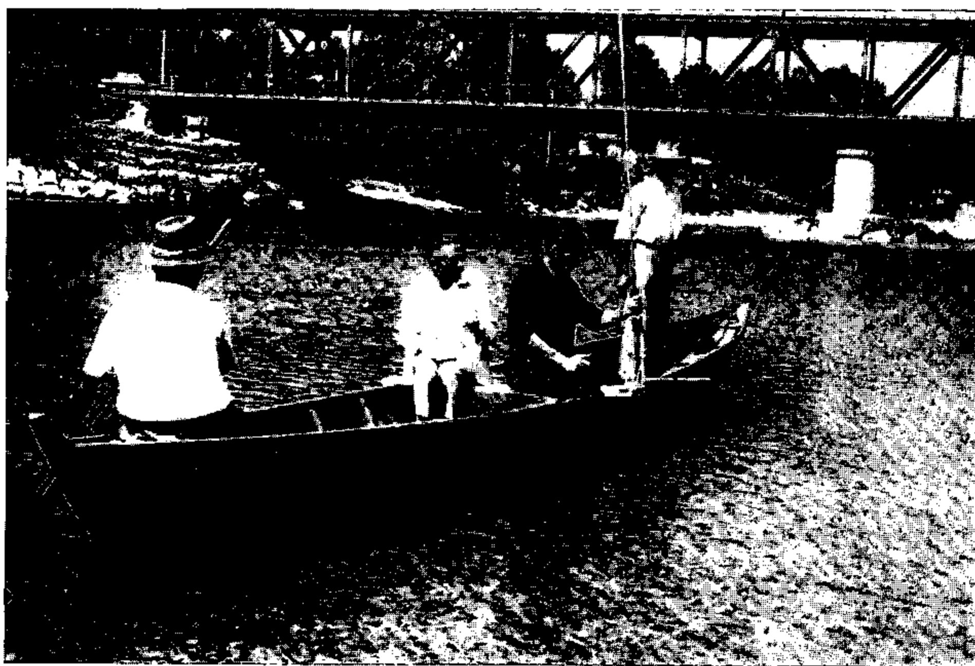
Misura di portata eseguita con barca
