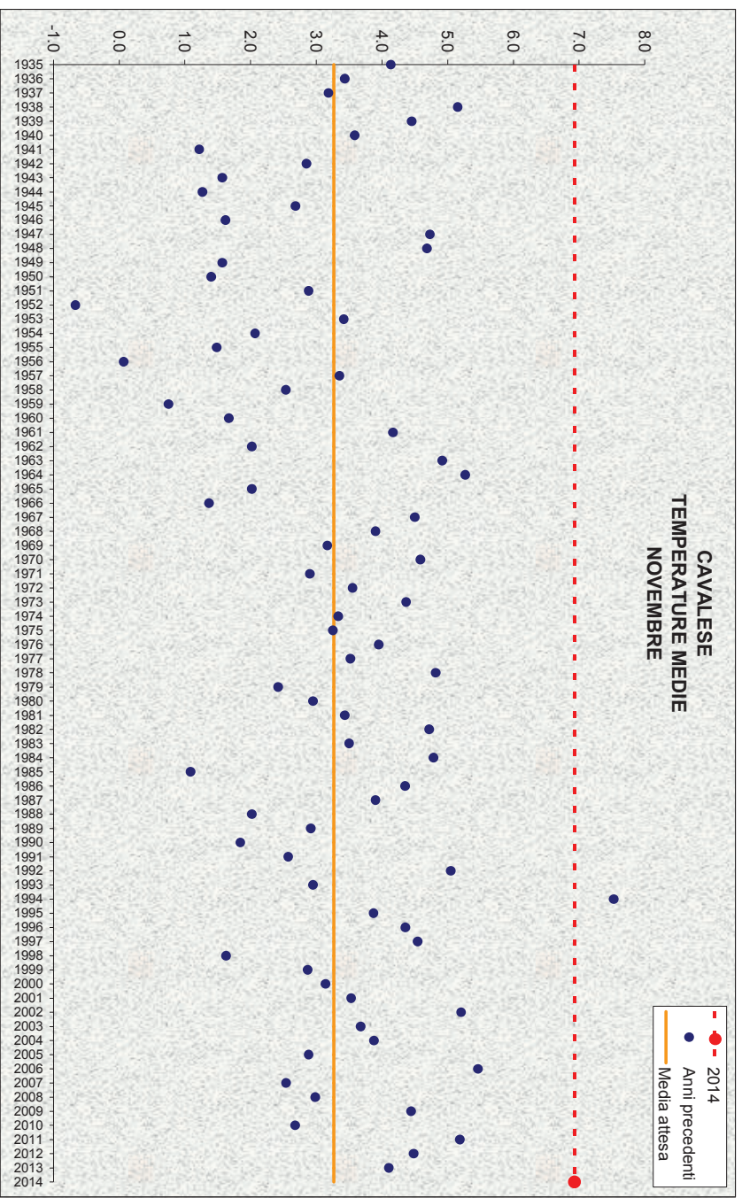
Figura 13: Temperature medie di novembre
