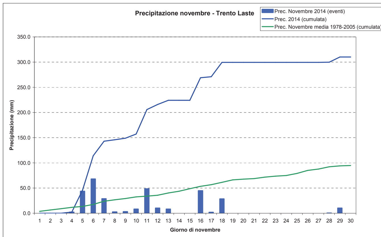
Figura 2: Precipitazioni giornaliera e cumulata di novembre
