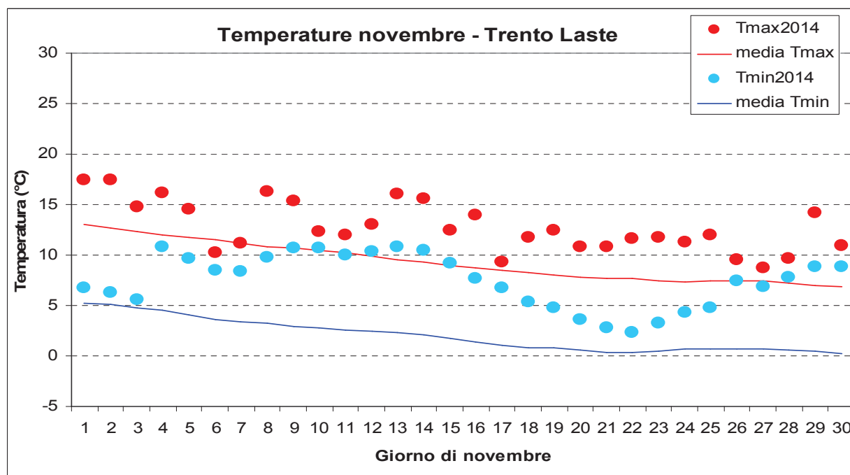
Figura 1: Temperature di novembre. La media delle Tmax e delle Tmin è riferita al periodo 1978-2005 (media mobile a 7 gg)
