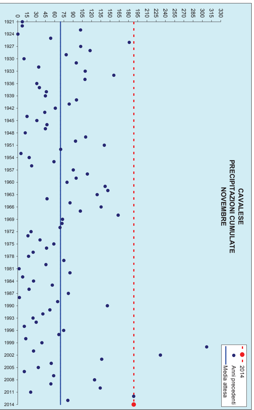
Figura 14: Precipitazioni di novembre
